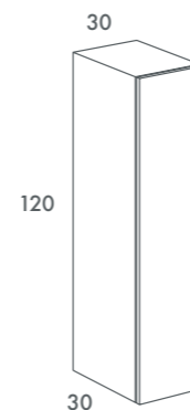
Estantería 2 estantes con puerta de 120 · Shelving with door of 120 2 shelf
